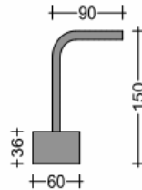
Listwa jedno rzętowa Ø 10mm
