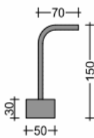
Listwa jedno rzętowa Ø 8mm
