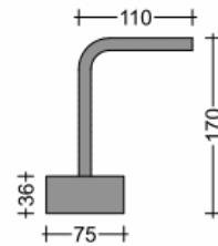
Listwa jedno rzętowa Ø 12mm
