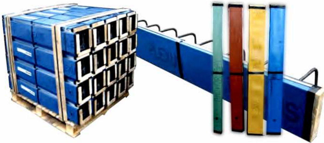
Listwa jedno rzętowa Ø 12mm
